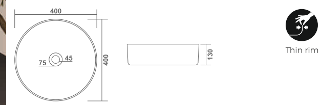
SPELL L 400 W 400 H 130mm L 16" W 16" H 5"
