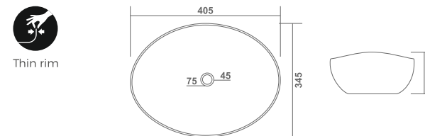
L 345 W 405 H 180mm L 14" W 16" H 7" ANTIQUÉ
