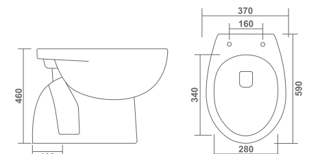
OZONE L 590 W 370 H 460mm
